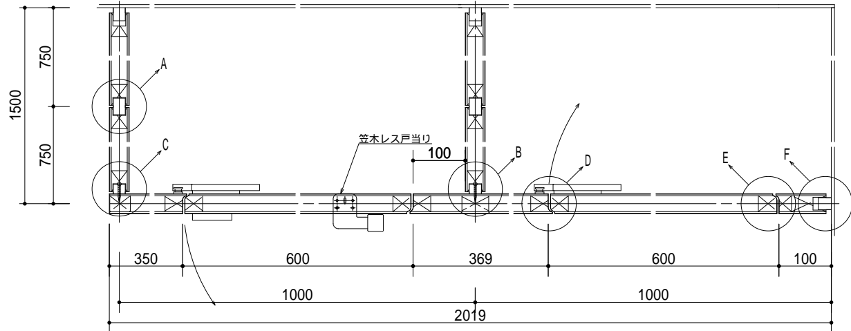
横方向断面図
