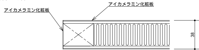
隔て納まり
