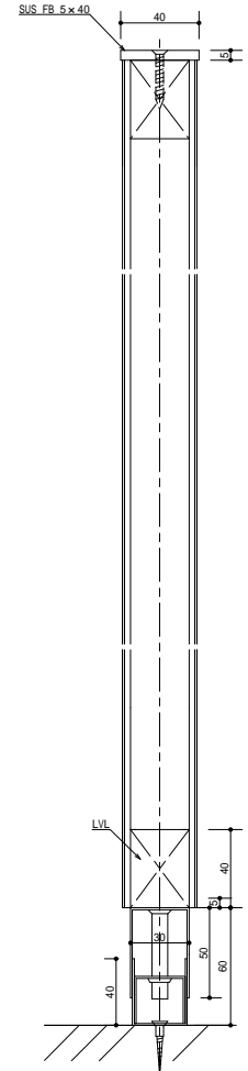
縦方向断面図 笠木仕様
