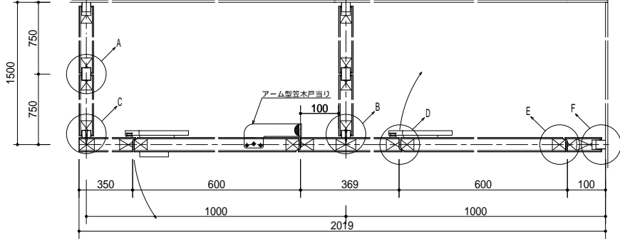
横方向断面図
