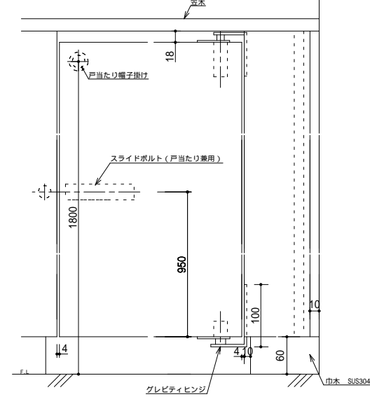
内開き仕様
