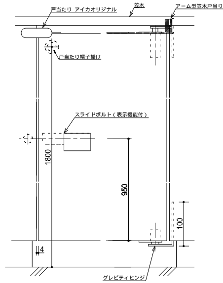
外開き仕様
