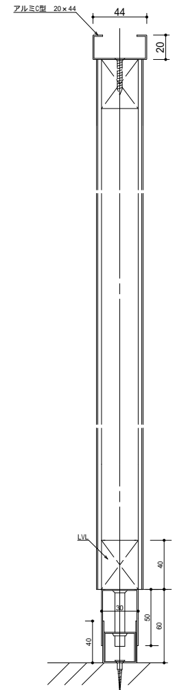
縦方向断面図 笠木仕様
