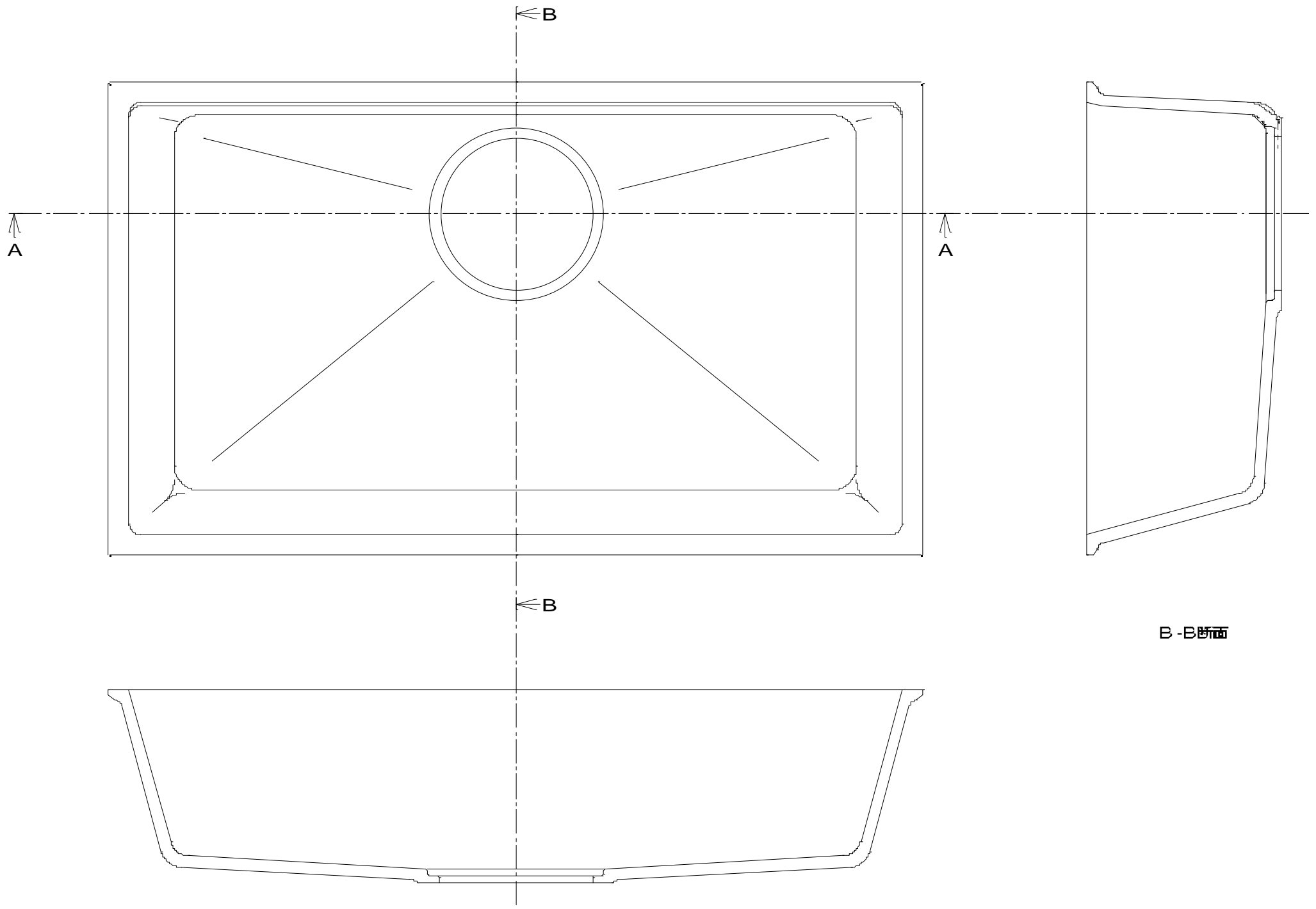
A-A断面
