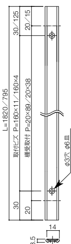
棚柱形状図
