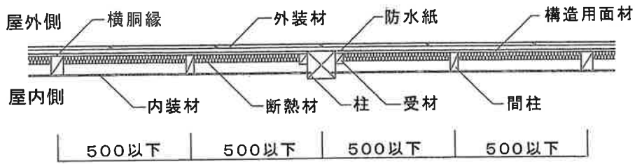
水平断面図[横胴縁、外装材縦張、真壁造(欠き込み)仕様]
