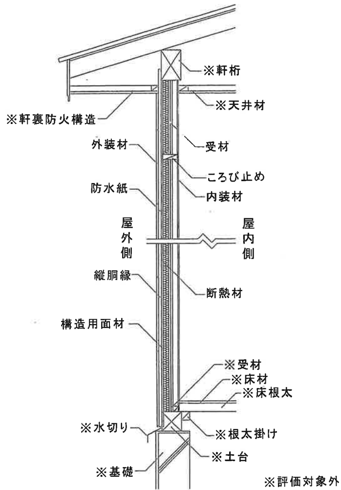
鉛直断面図[縦胴縁、外装材横張、真壁造(受材)仕様]
