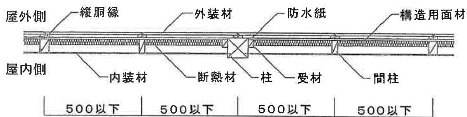
水平断面図[縦胴縁、外装材縦張、真壁造(欠き込み)仕様]
