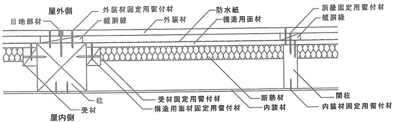
水平断面図[縦胴縁、外装材横張、大壁造仕様]
