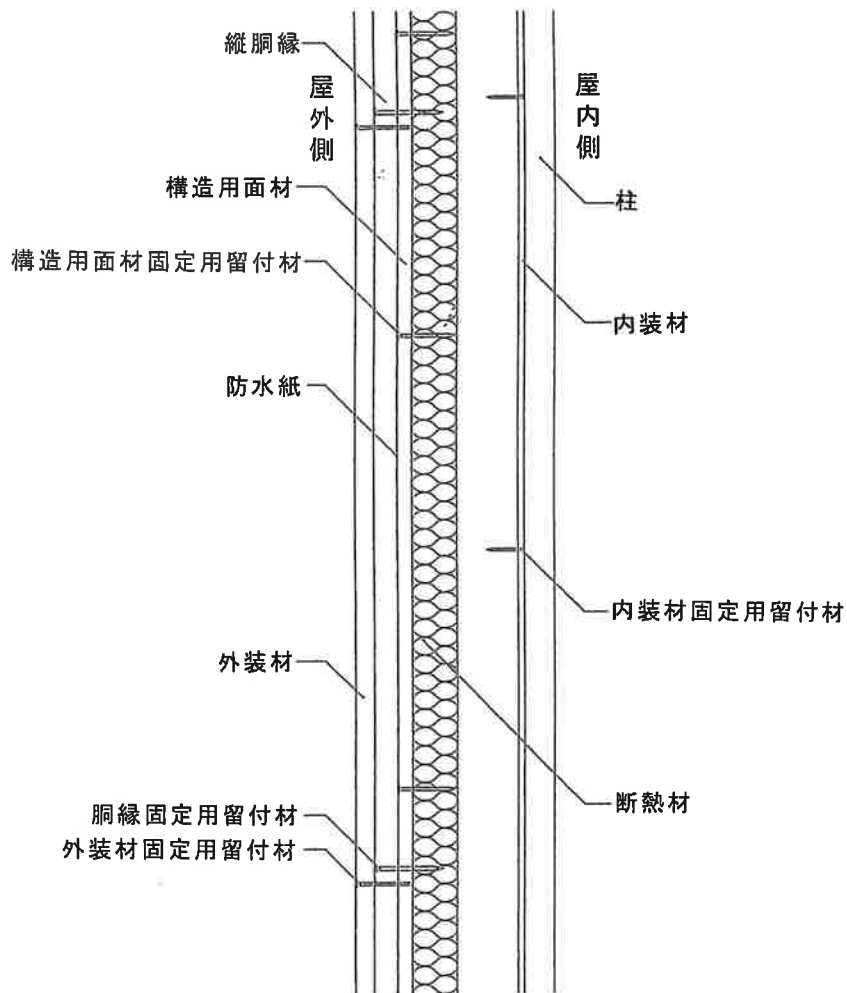
鉛直断面図[縦洞縁、外装材縦張、真壁造(欠き込み)仕様]
