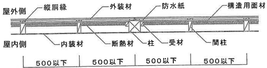
水平断面図 [縦胴縁、外装材横張、大壁造仕様]
