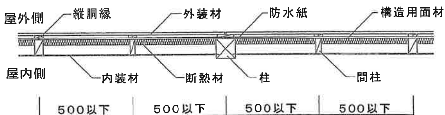
水平断面図[縦胴縁、外装材横張、真壁造(欠き込み)仕様、 構造用面材が柱を覆う場合(受材なしの場合)]
