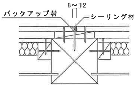
③バックアップ材+シーリング目地
