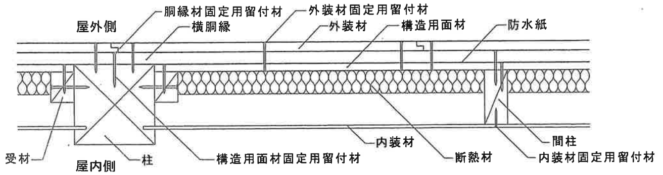
水平断面図[横洞縁、外装材縦張、真壁造(欠き込み)仕様]
