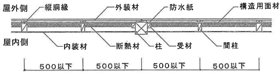
水平断面図[縦胴縁、外装材横張、真壁造(欠き込み)仕様]
