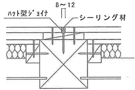
②ハット型ジョイナー+シーリング目地
