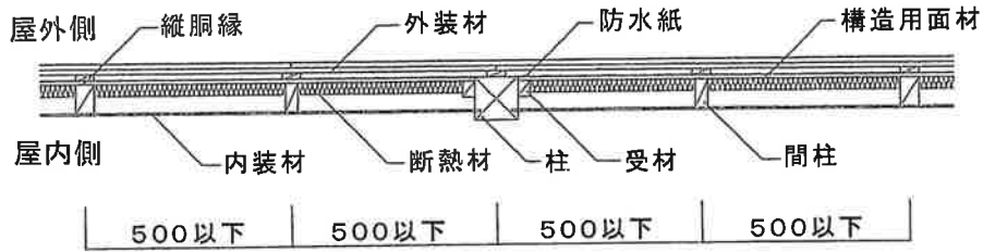
水平断面図[縦胴縁、外装材よろい張、真壁造(欠き込み)仕様]
