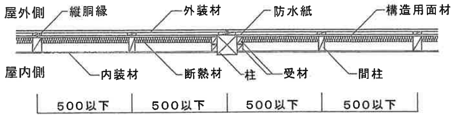
水平断面図[縦胴縁、外装材横張、真壁造(受材)仕様]
