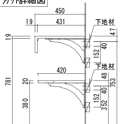
フ ラケット詳細図
