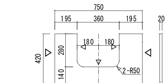
固定棚平面图
