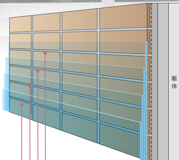
■ 施工断面図
