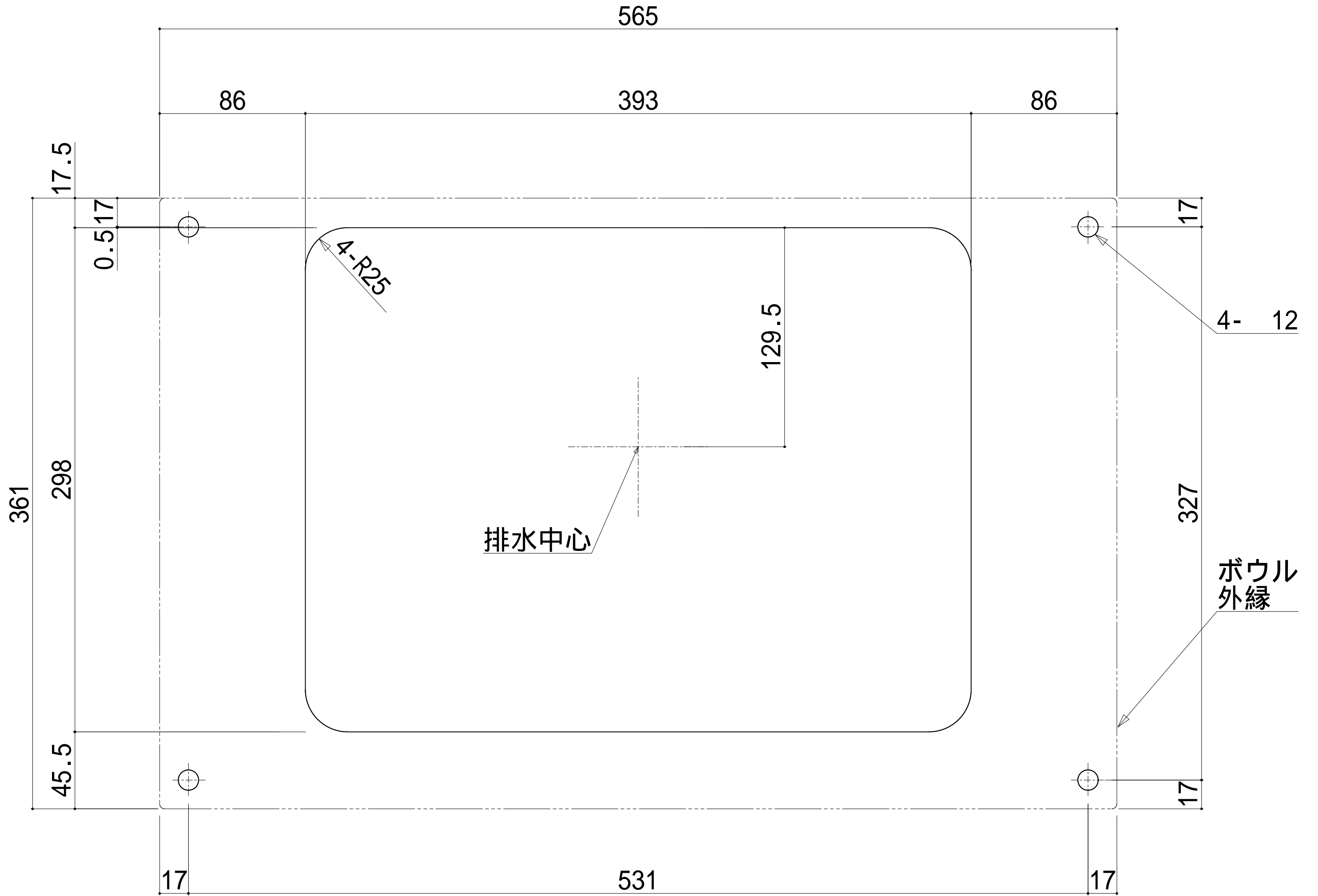
『 K M C 7 * * * * - 3 A オンボウル用穴加工図(縮尺:1/2) 』
